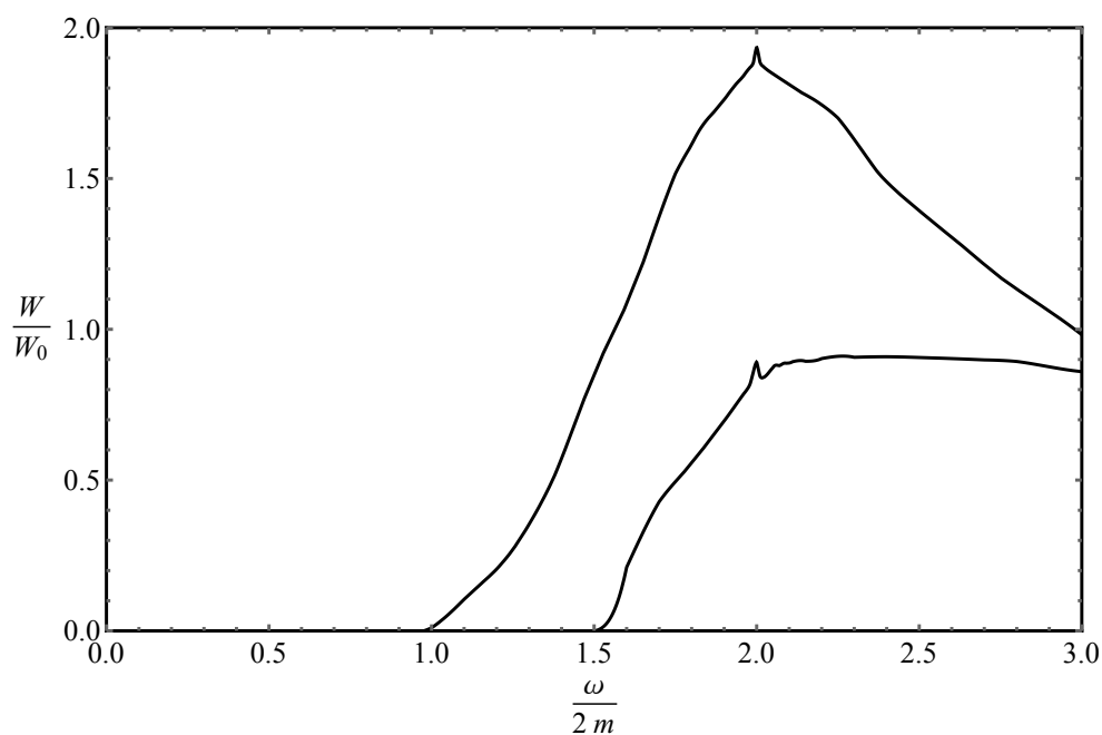
Рис. 3.7. Коэффициент поглощения фотона в канале \gamma_1 \rightarrow \gamma_2\gamma_2 для значений магнитного поля B/B_e = 100 (верхняя кривая), B/B_e = 200 (нижняя кривая) Здесь W_0 = (\alpha/\pi)^3 m \simeq 3.25 \cdot 10^2 \text{см}^{-1} .
