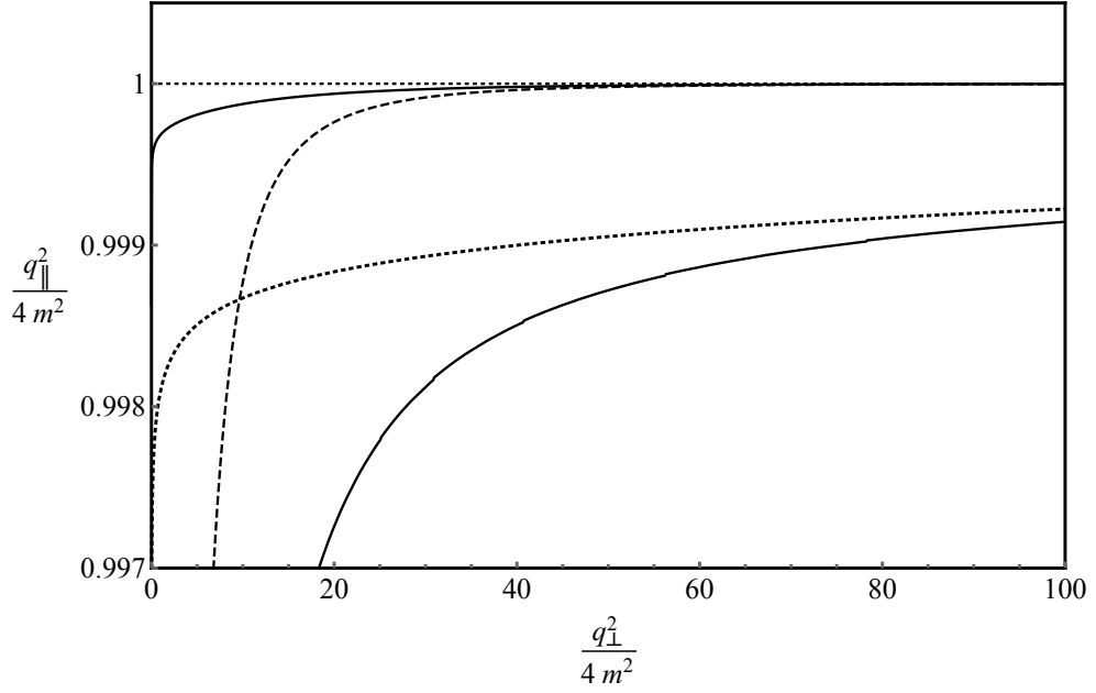
Рис. 3.3. Закон дисперсии для фотона второй моды с учётом вклада связанной e^+e^- -пары в сильном магнитном поле, B = 200B_e . Пунктирная кривая - спектральная линия фотона без учёта вклада позитрония, точечная кривая – спектральная линия позитрония.
