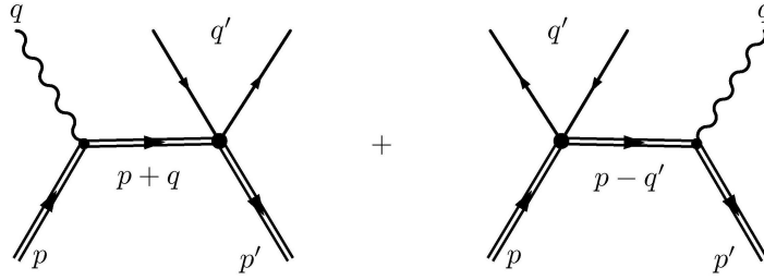
Рис. 2.1. Диаграммы Фейнмана для реакции \gamma e \rightarrow e\nu\bar{\nu} . Двойные линии обозначают, что влияние внешнего поля на начальное и конечное состояние и на элеткронный пропагатор учтено точно.
