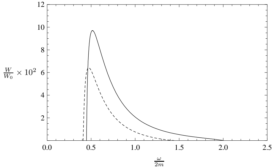
Рис. 3.4. Вероятность расщепления фотона по каналу \gamma_2 \rightarrow \gamma_1\gamma_1 в сильном магнитном поле ( B/B_e = 200 ) и холодной ( T = 50 кэВ) плазме при химическом потенциале 1 МэВ (сплошная линия) и 0.75 МэВ (штриховая линия). Здесь \theta = \pi/2 , W_0 = (\alpha/\pi)^3 m \simeq 3.25 \cdot 10^2 \text{см}^{-1}
