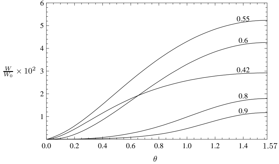
Рис. 3.5. Зависимость вероятности расщепления фотона по каналу \gamma_2 \rightarrow \gamma_1\gamma_1 от угла между импульсом начального фотона и направлением магнитного поля при различных энергиях начального фотона ( B/B_e = 200 , T = 50 кэВ, \mu = 0.75 МэВ). Числа на кривых соответствуют отношению \omega/2m . W_0 = (\alpha/\pi)^3 m \simeq 3.25 \cdot 10^2 \text{см}^{-1}
