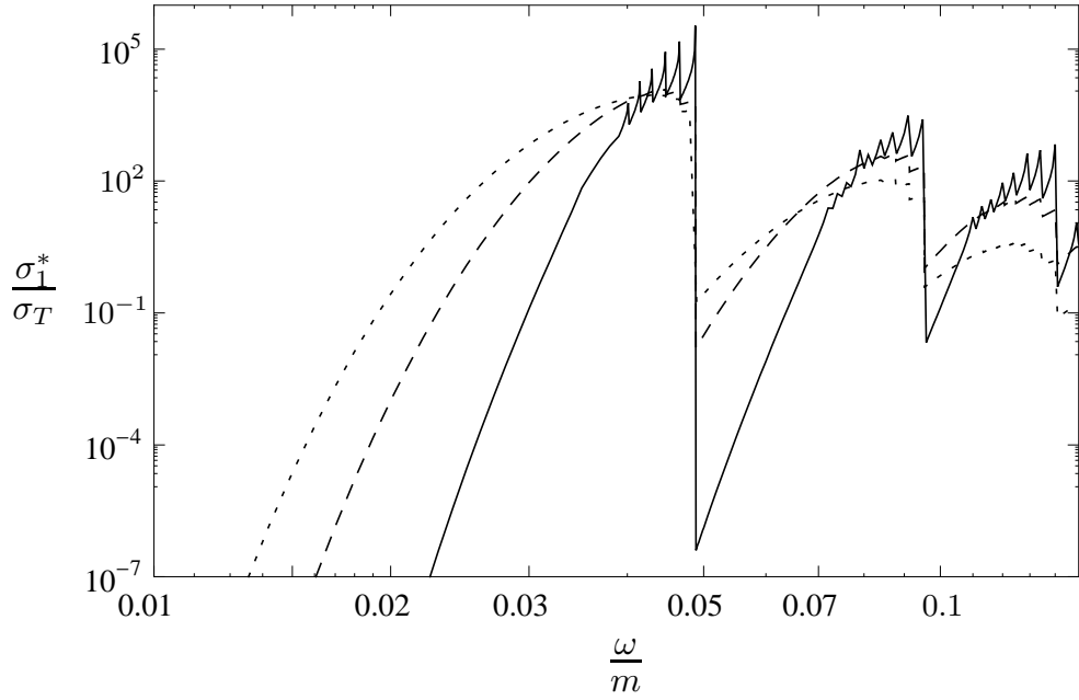
Рис. 2.3. Сечение (в единицах \sigma_T ) рассеяния фотона моды 1, \gamma^{(1)}e \rightarrow e , в сильном магнитном поле B = 5 \times 10^{12} Гс, проинтегрированное по начальным электронам с функцией распределения f_{E_e} при T = 20 кэВ и \mu = 0 , как функция энергии (в единицах массы электрона) фотона для различных значений углов между импульсом фотона и направлением магнитного поля: \theta = 90^\circ – сплошная кривая, \theta = 60^\circ – пунктирная кривая, \theta = 30^\circ – точечная кривая.
