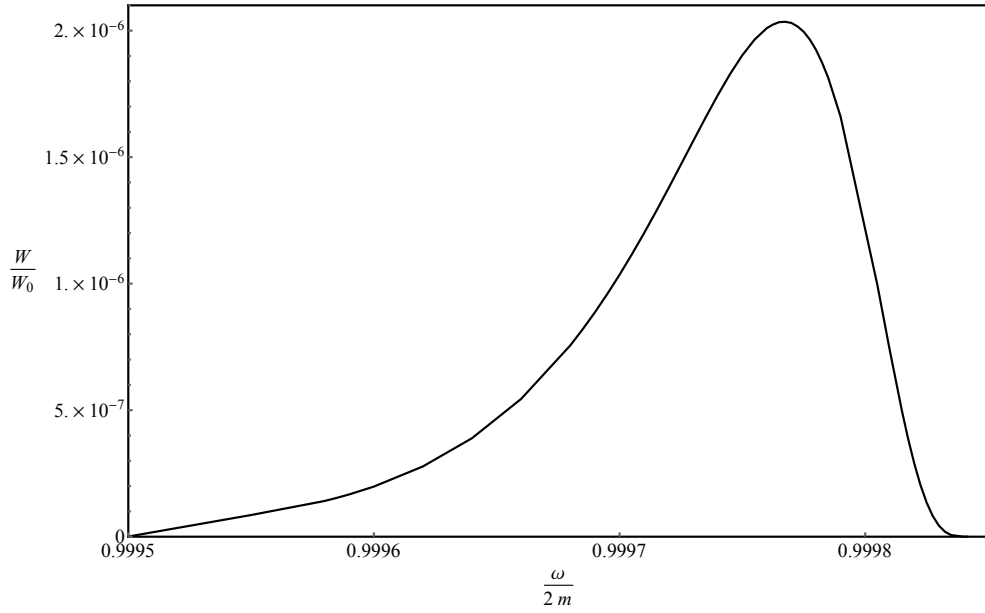
Рис. 3.10. Коэффициент поглощения фотона в канале \gamma_2 \rightarrow \gamma_1\gamma_1 в сильном магнитном поле ( B/B_e = 200 ). W_0 = (\alpha/\pi)^3 m \simeq 3.25 \cdot 10^2 \text{см}^{-1} .
