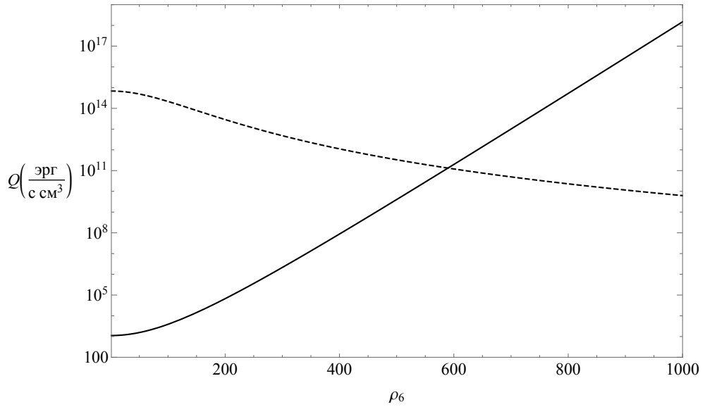
Рис. 2.2. Зависимость светимости фотонейтринного процесса от плотности плазмы для значений параметров B = 50B_e и T = 10^9 \text{ К} . Сплошная линия соответствует светимости резонансного процесса, пунктирная – без учёта резонанса.
