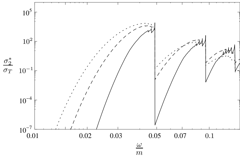
Рис. 2.4. Сечение (в единицах \sigma_T ) рассеяния фотона моды 2, \gamma^{(2)}e \rightarrow e , в сильном магнитном поле B = 5 \times 10^{12} Гс, проинтегрированное по начальным электронам с функцией распределения f_{E_e} при T = 20 кэВ и \mu = 0 , как функция энергии (в единицах массы электрона) фотона для различных значений углов между импульсом фотона и направлением магнитного поля: \theta = 90^\circ – сплошная кривая, \theta = 60^\circ – пунктирная кривая, \theta = 30^\circ – точечная кривая.
